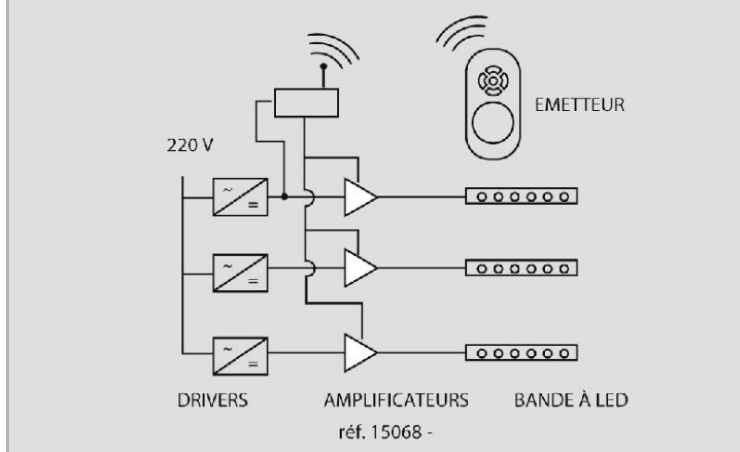
Schéma général de plusieurs drivers avec le même contrôleur
